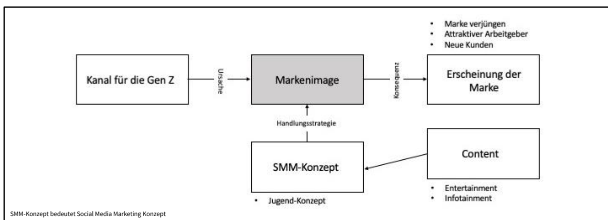
Abbildung 5: Rahmenmodell 2 – Markenimage
