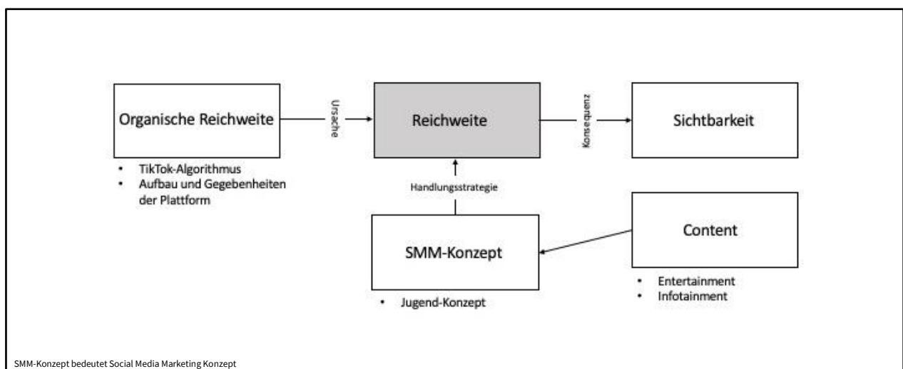
Abbildung 6: Rahmenmodell 3 – Reichweite
