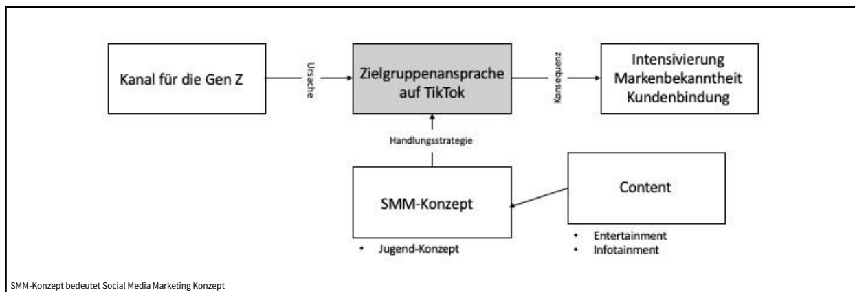
Abbildung 4: Rahmenmodell 1 - Zielgruppenansprache
